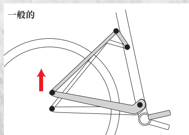
ピボット位置が低いと振り子の原理により真上に衝撃がいきます。
