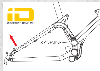
i-DRIVEのピボット位置は高いので衝撃を斜め後方に受け流します。
