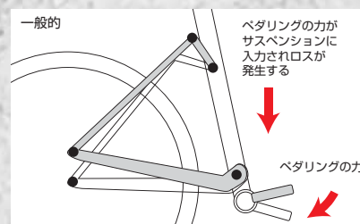
BBがフロントフレームに接続されているとベダリングの力がサスペンションに入力され、常にロスが発生し続けます。
