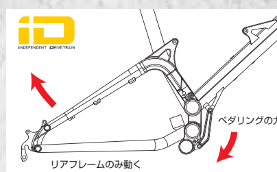
i-DRIVEではBBがリアにフローティング方法で接続されているのでロスの発生が極めて少ない。
