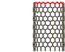
単層カーボンノチューブの構造 ほとんどの部分が蜂の巣状の六員環になっているが、五員環や七員環（赤色）の部分が存在し、これによって単なる円筒ではない構造を作り得る。
