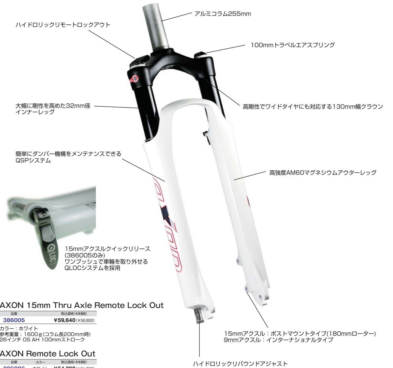
ワンタッチでスルーアクスルの車輪を取り外せるQLOCシステム
